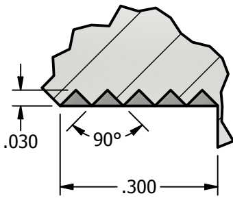
DETAIL D1
