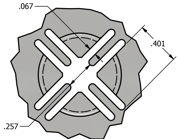
DETAIL D1
