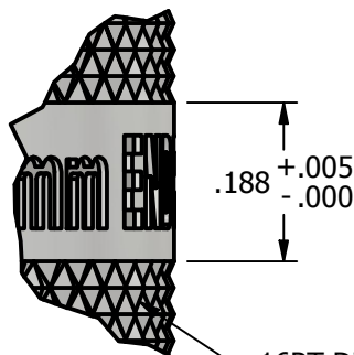
DETAIL D2
